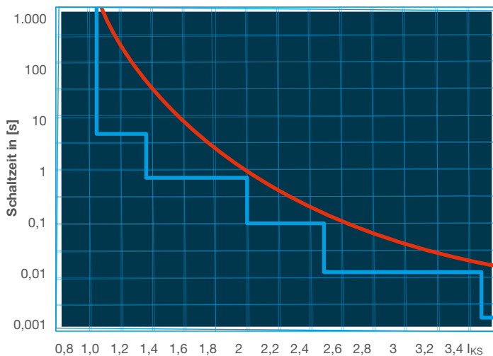
Vielfache des Nennstromes/Bemessungsstrom // Kennlinie REX12
